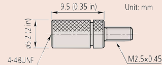
21AAA012 Adaptér pro úchylkoměry EN ISO (metrické) závit 4-48 UNF
