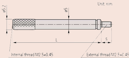
A = M 2,5 x 0,45 mm (metrický)
