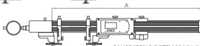
RANGE SPRING SYSTEM 20 MM. INSIDE/OUTSIDE CORSO UTILE PRECARICA 20 MM. INTERNO/ESTERNO
