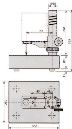
957460 Měřicí stojan
