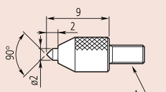
Kuželový dotek tvrdokový (120057D)
